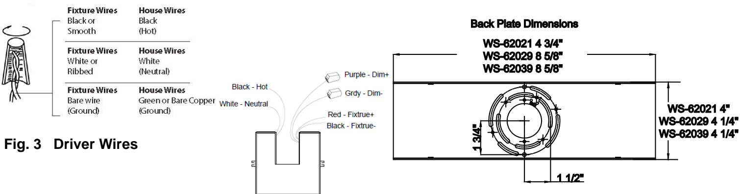
Fig. 2 Wiring
